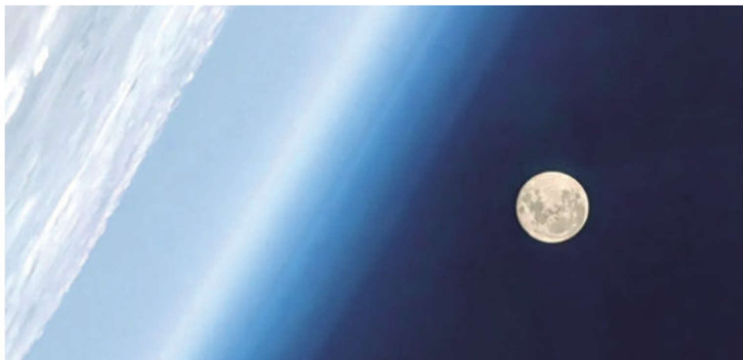
神舟十四号航天员陈冬在轨拍摄的地球、月球 中国载人航天工程办公室提供
