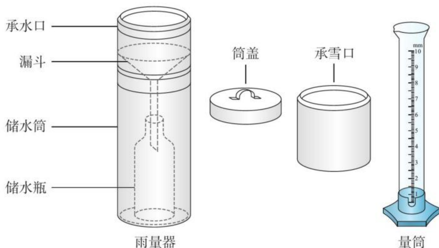
图4.17 雨量器和配套量筒
