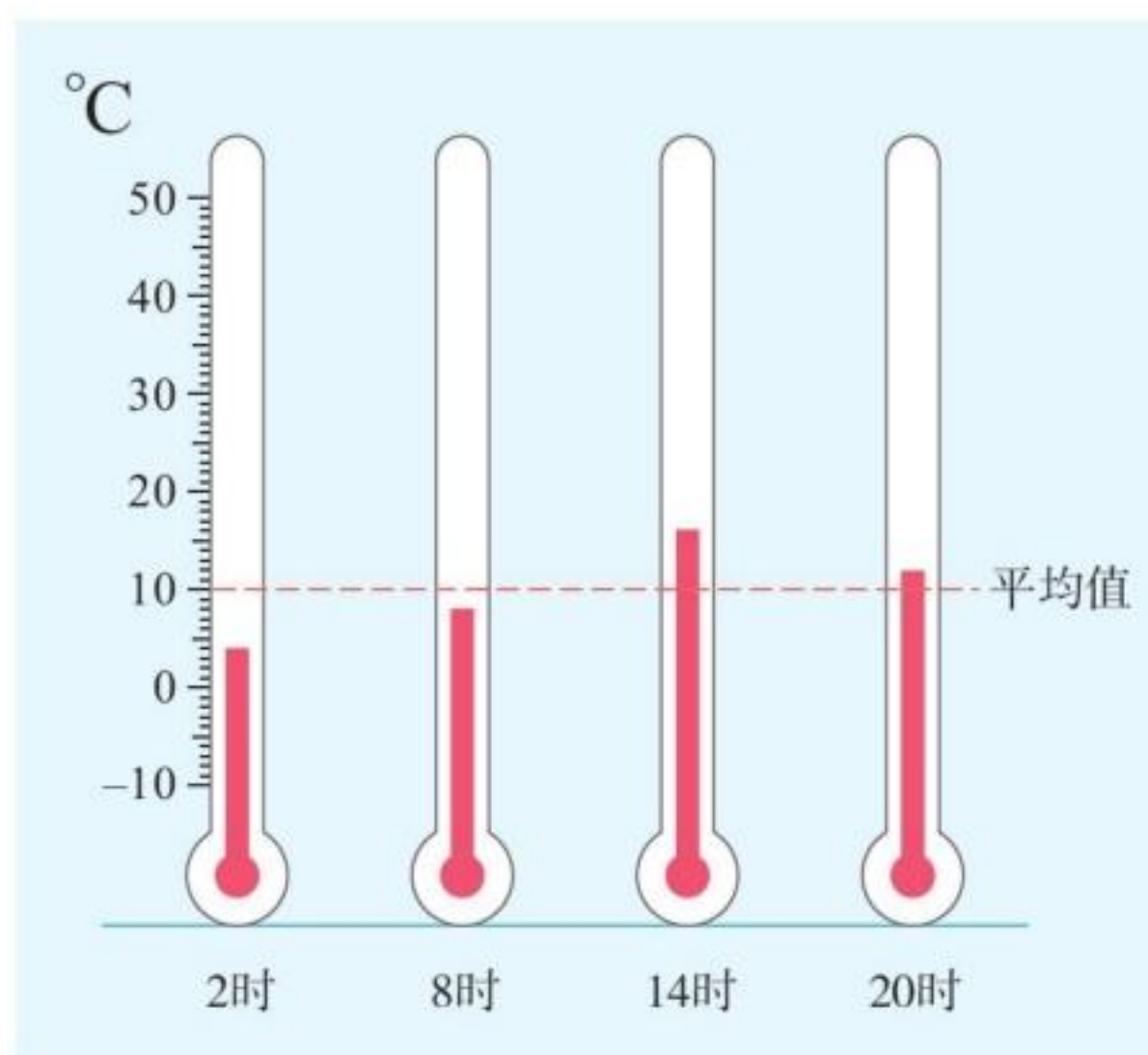
图4.7 日平均气温计算示意
