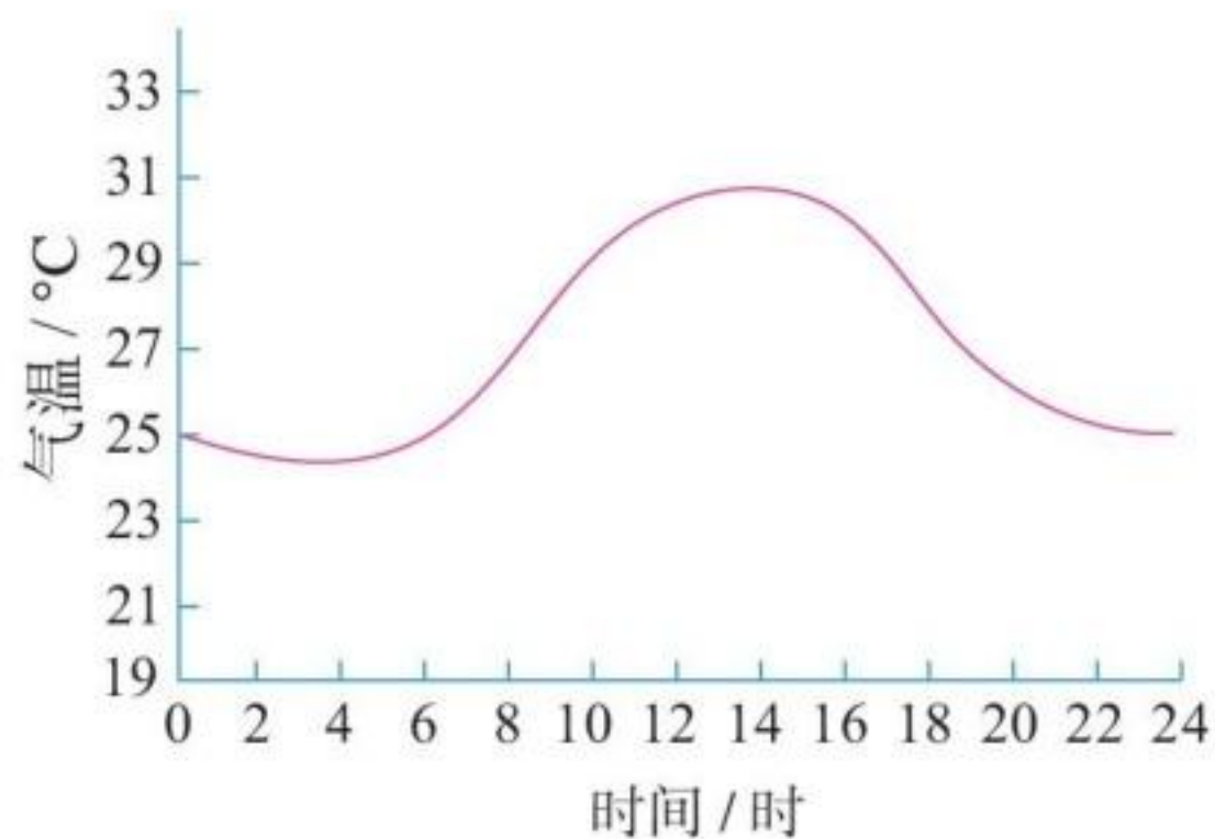
图4.8 气温日变化
