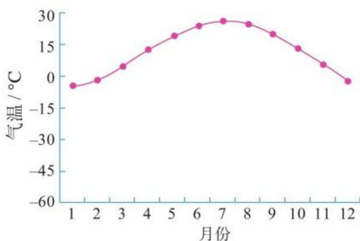
图4.9 气温年变化
