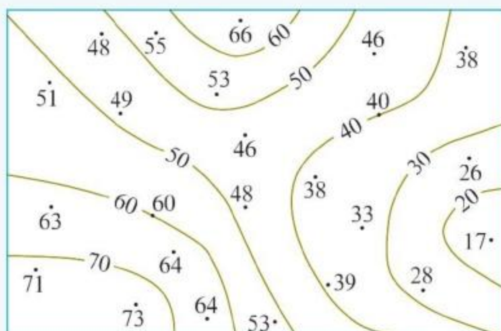
图2.12 等高线的绘制
