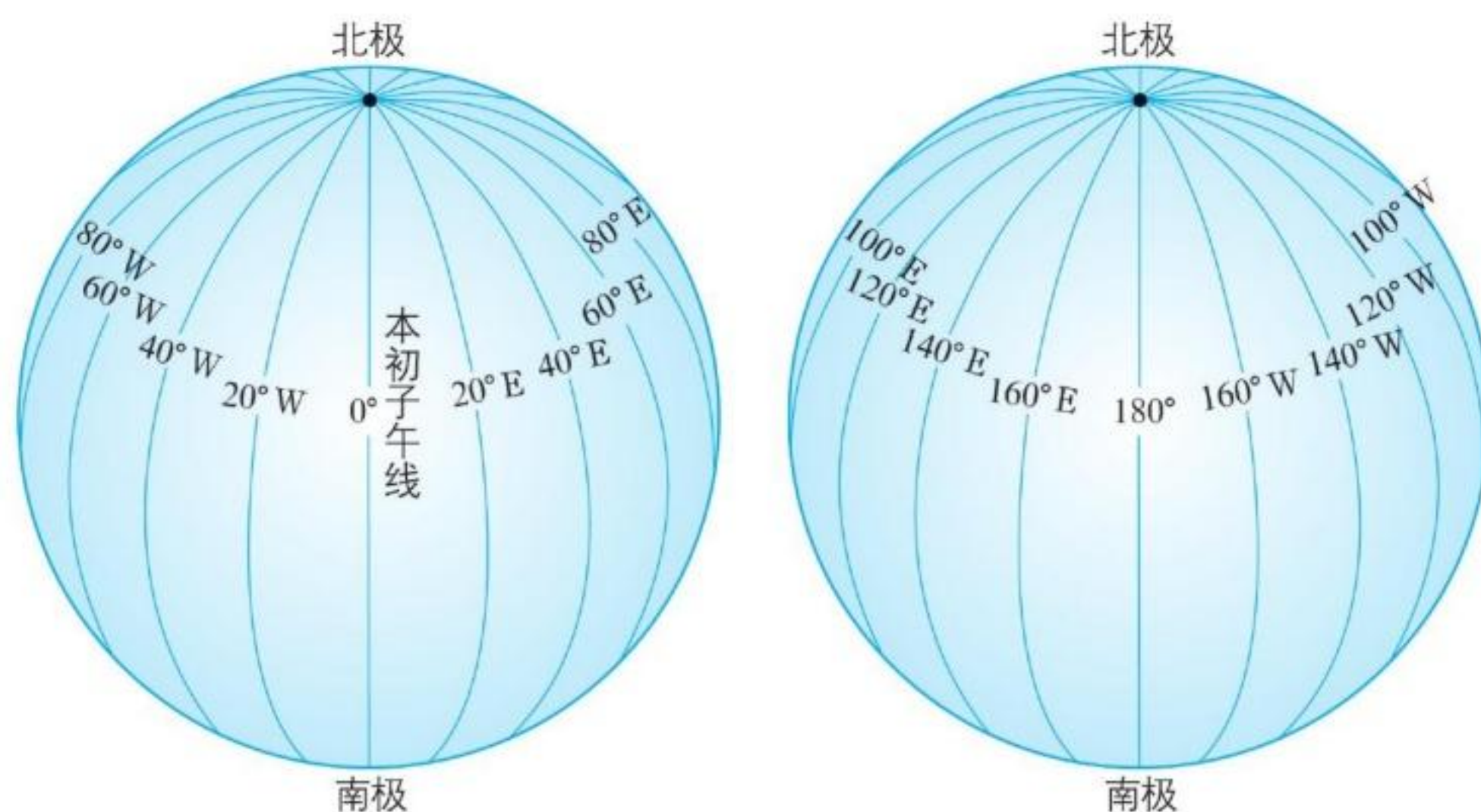
图 1.11 经线和经度
