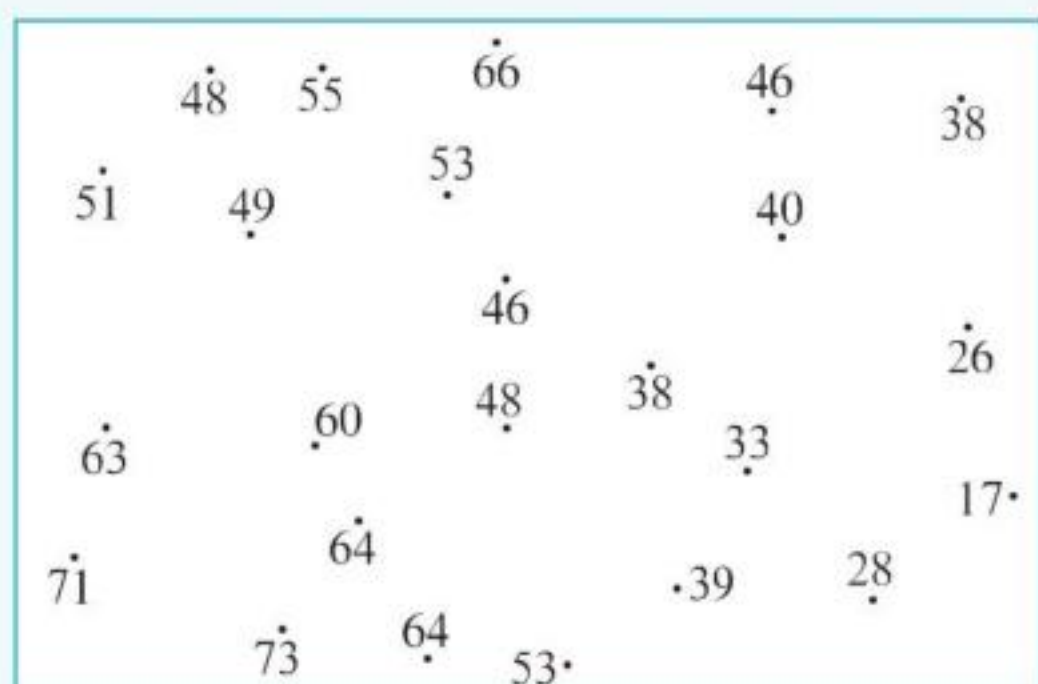
图2.11 测绘点海拔的标注
