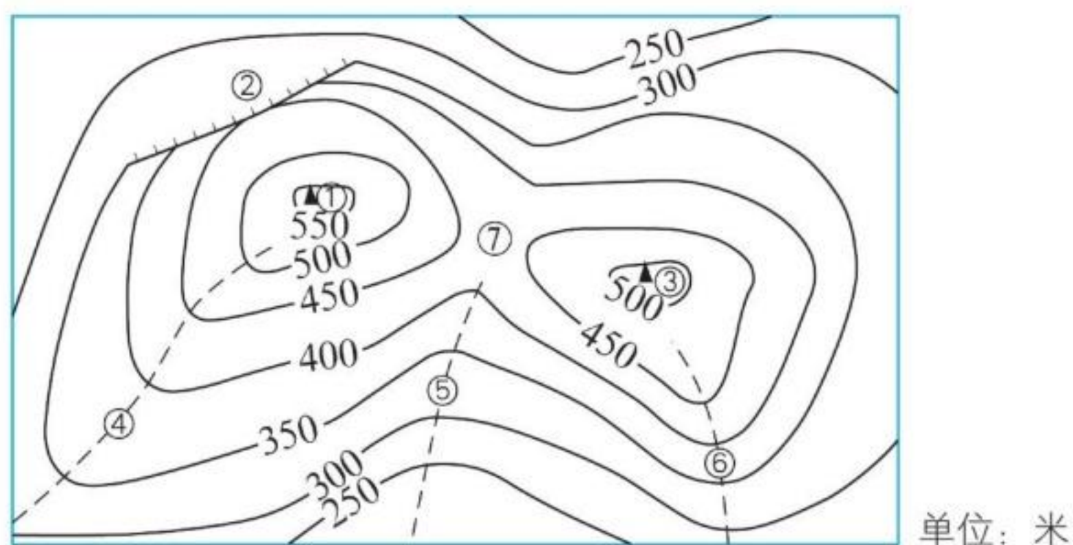
图 2.13 等高线地形图
