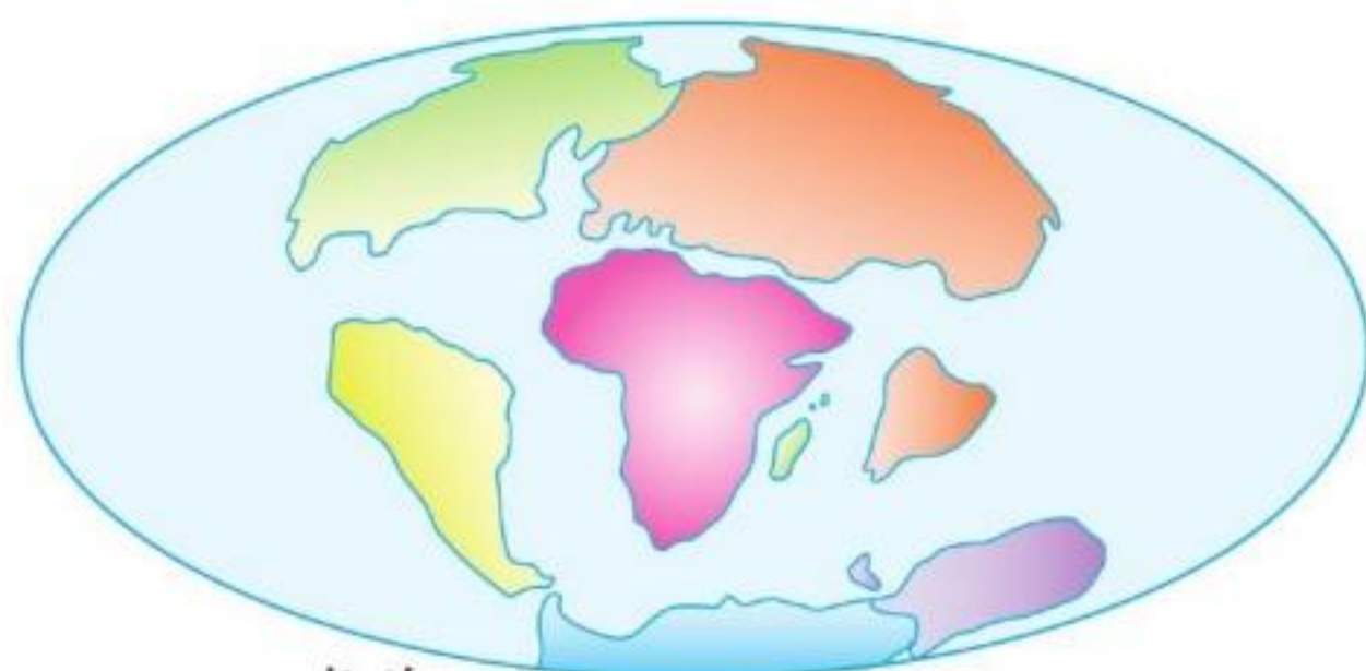
6 500 万年前
