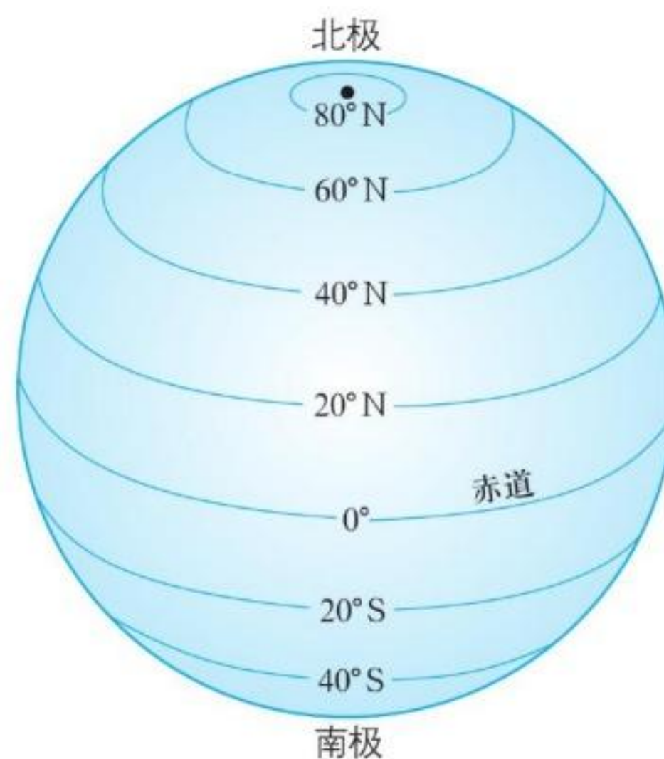
图1.15 纬线和纬度
