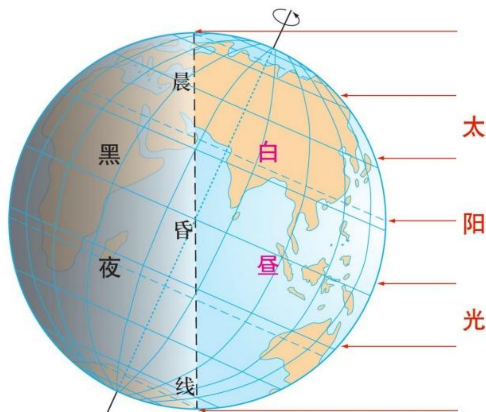
图1.18 昼与夜
