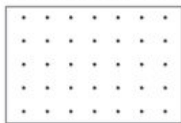
等腰三角形
