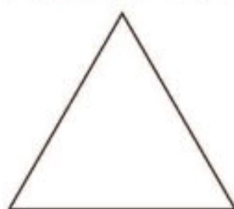
等边三角形
