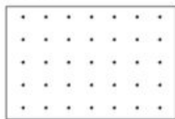
钝角三角形
