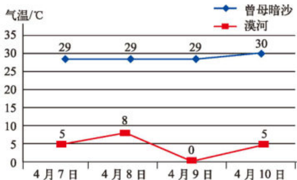
4月7~10日我国南北两地最高气温统计图
