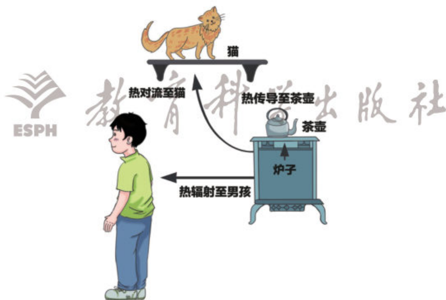
三种热传递方式
