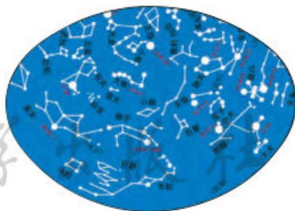
统一的星座图
