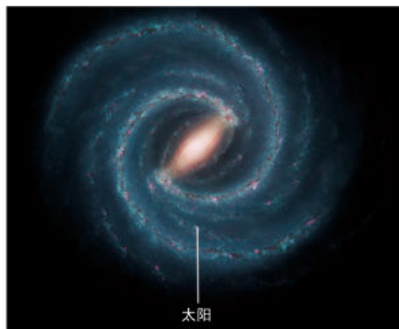
银河系的“俯视图”
