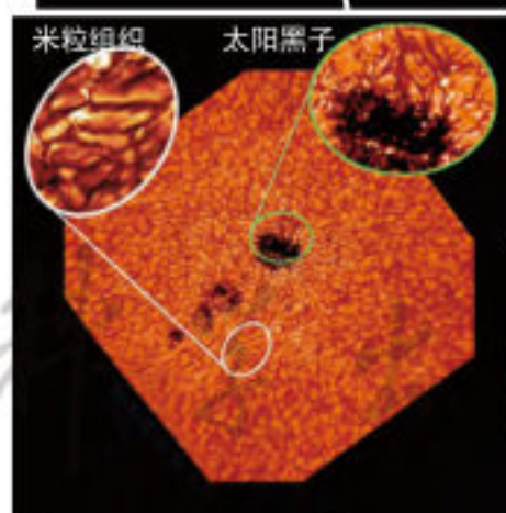
太阳光球上的米粒组织
