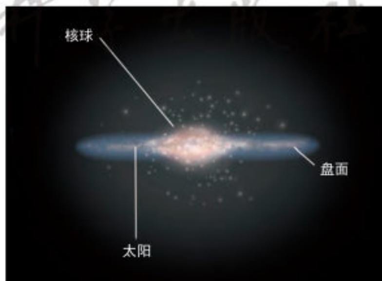
银河系的“侧视图”
